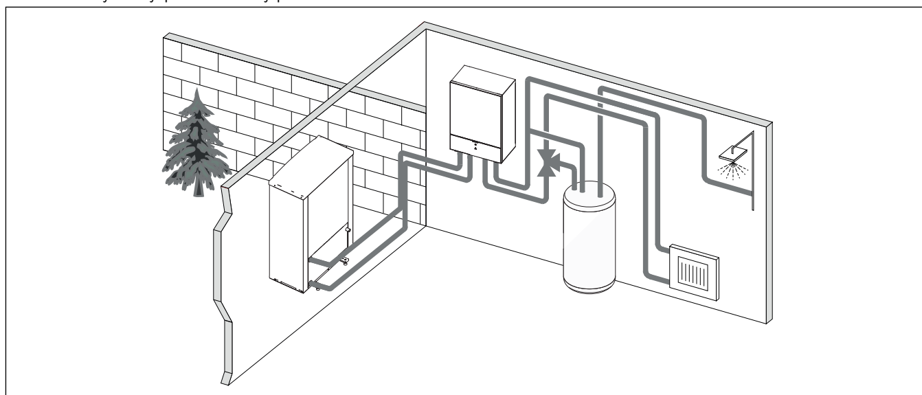
Рис. 3 Тепловой насос Compress 7000i AW, внутренний блок AWE с дополнительным электронагревателем и внешним баком-водонагревателем
