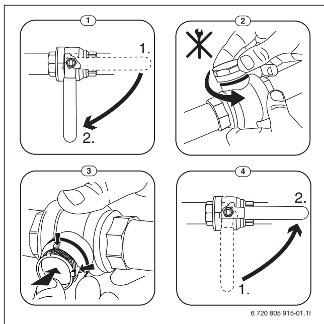
Рис. 8 Чистка сетчатого фильтра
