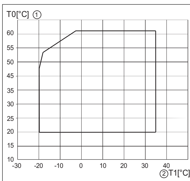
Рис. 1 Тепловой насос без дополнительного нагревателя
