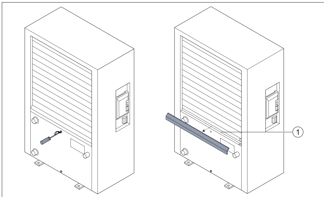
Рис. 9 Конденсатная ванна теплового насоса
