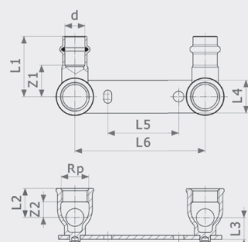
Монтажный узел Sanpress Модель 2222.2
