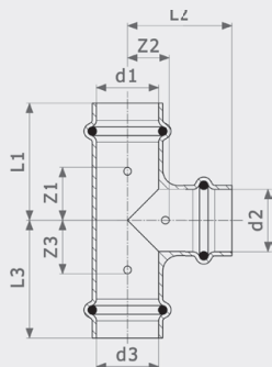
Тройник Profipress - медь Модель 2418
