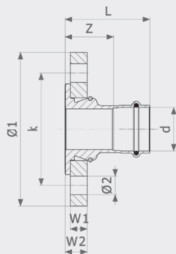
Фланцевый переход Sanpress - ! Модель 2259.5
