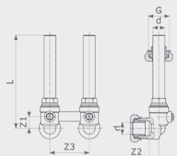
Соединительный комплект для подключения радиатора - бронза никелированная матовая Модель 1097.7
