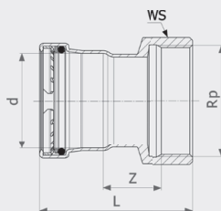
Соединительный элемент Profipress XL - медь Модель 2412XL
