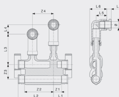
Подключение радиаторов при плитусной разводке - бронза Модель 2277.2
