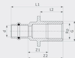
Водорозетка Sanpress - ! Модель 2232.3
