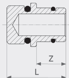
Соединительный элемент переходной - латунь Модель 2233.6
