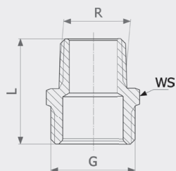
Комплект переходников - бронза никелированная матовая Модель 1022.6
