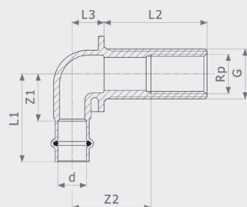
Водорозетка Sanpress - ! Модель 2232.1
