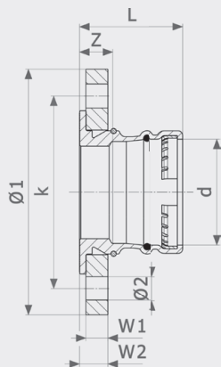
Фланцевый переход Sanpress XL - бронза Модель 2259.5XL
