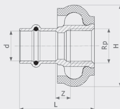
Соединительный элемент Sanpress - ! Модель 2212.4
