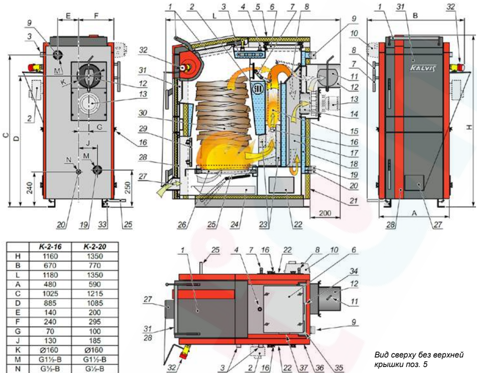
Рис. 1. Конструкция котла.
